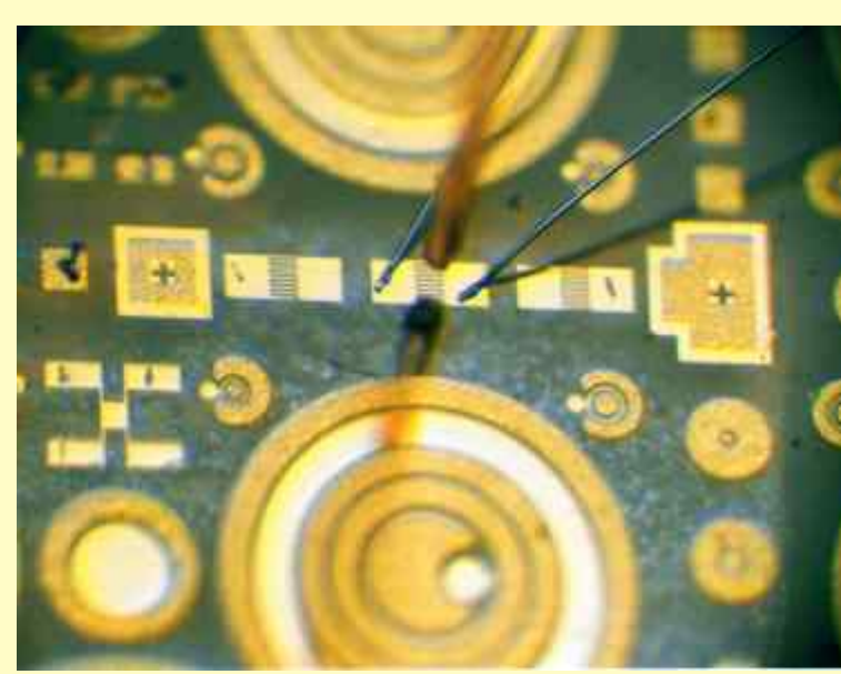
GaN HFETs test structure
